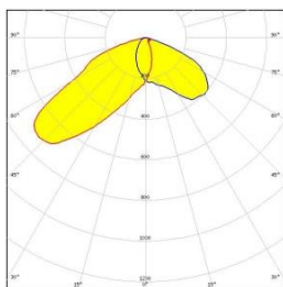
5144 - levostranná
